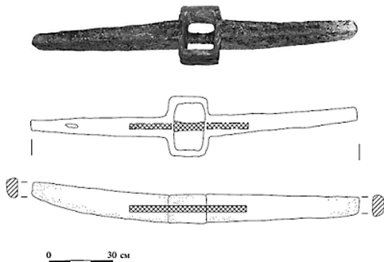
Рис. 7. Свинцовый шток типа III (сост. по: [3, с. 133])
