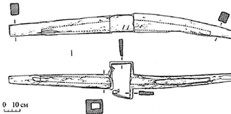
Рис. 5. Свинцовый шток типа IIIA (сост. по: Лысенко А. В., Герасимов В. Е. О находках штоков античных якорей у мыса Плака в Крыму // Российская археология. 2008. №3. С. 122)
