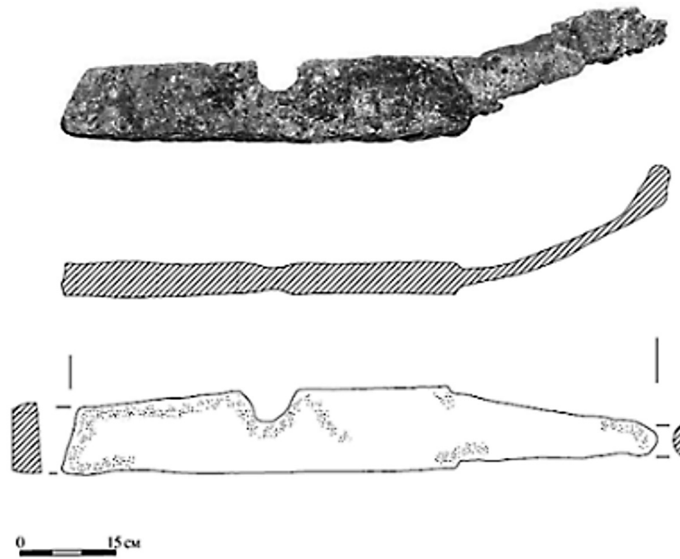
Рис. 4. Плечо свинцового штока типа IV (сост. по: [3, с. 114])
